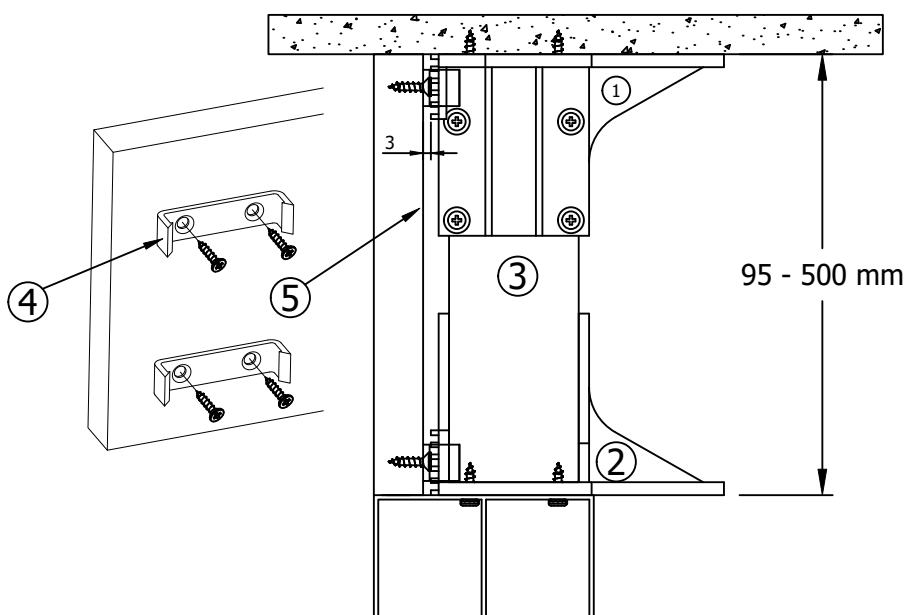
Figure A : Imposte au dessus du rail
