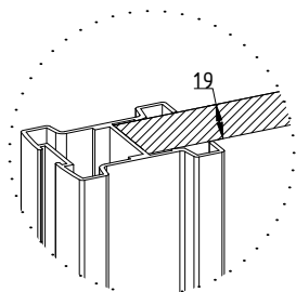
Panneau : épaisseur 19 mm
