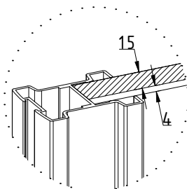
Vitre/Miroir : épaisseur 4 mm Panneau : épaisseur 15 mm
