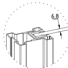
Vitre feuilletée : épaisseur 6,8 mm + réducteur
