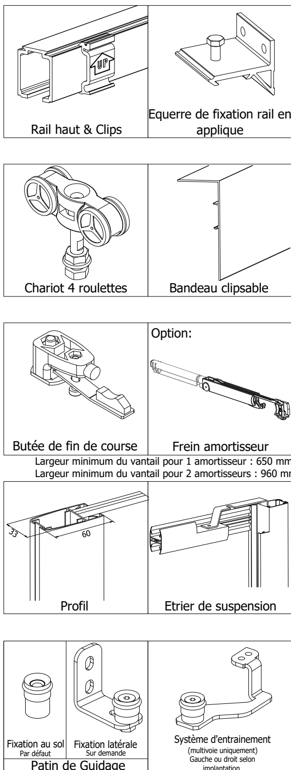
VUE DES ÉLÉMENTS
