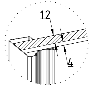
Vitre/Miroir : épaisseur 4 mm Panneau : épaisseur 12 mm
