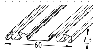
Rail Bas Acier laqué
