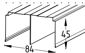
Rail Haut: -Acier laqué ou enrobé -Longueur maxi : 5450 mm
